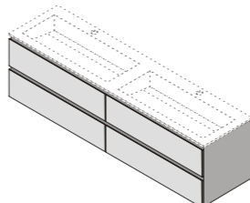
WD2218-0 W1800xD460xH500mm
